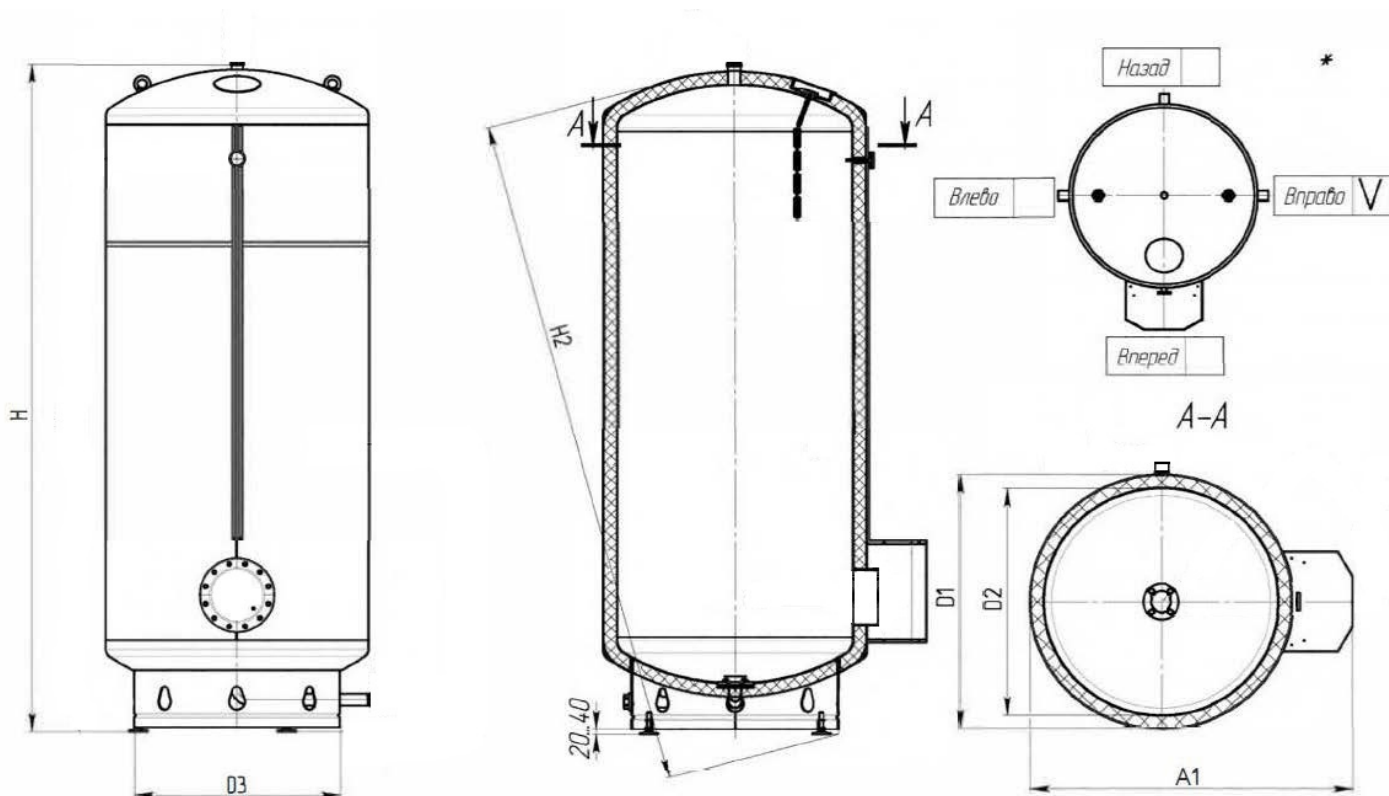
Рис. 2 Размеры основные
