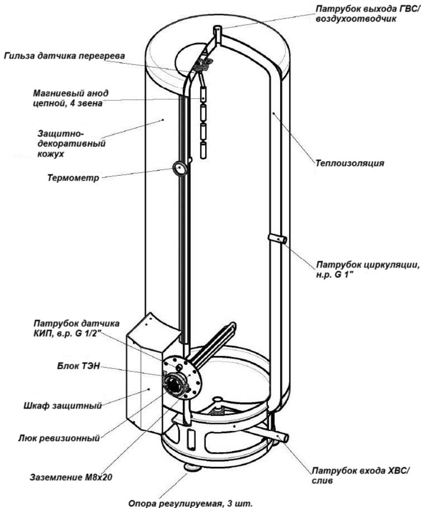
Рис. 1 Общий вид бойлера
