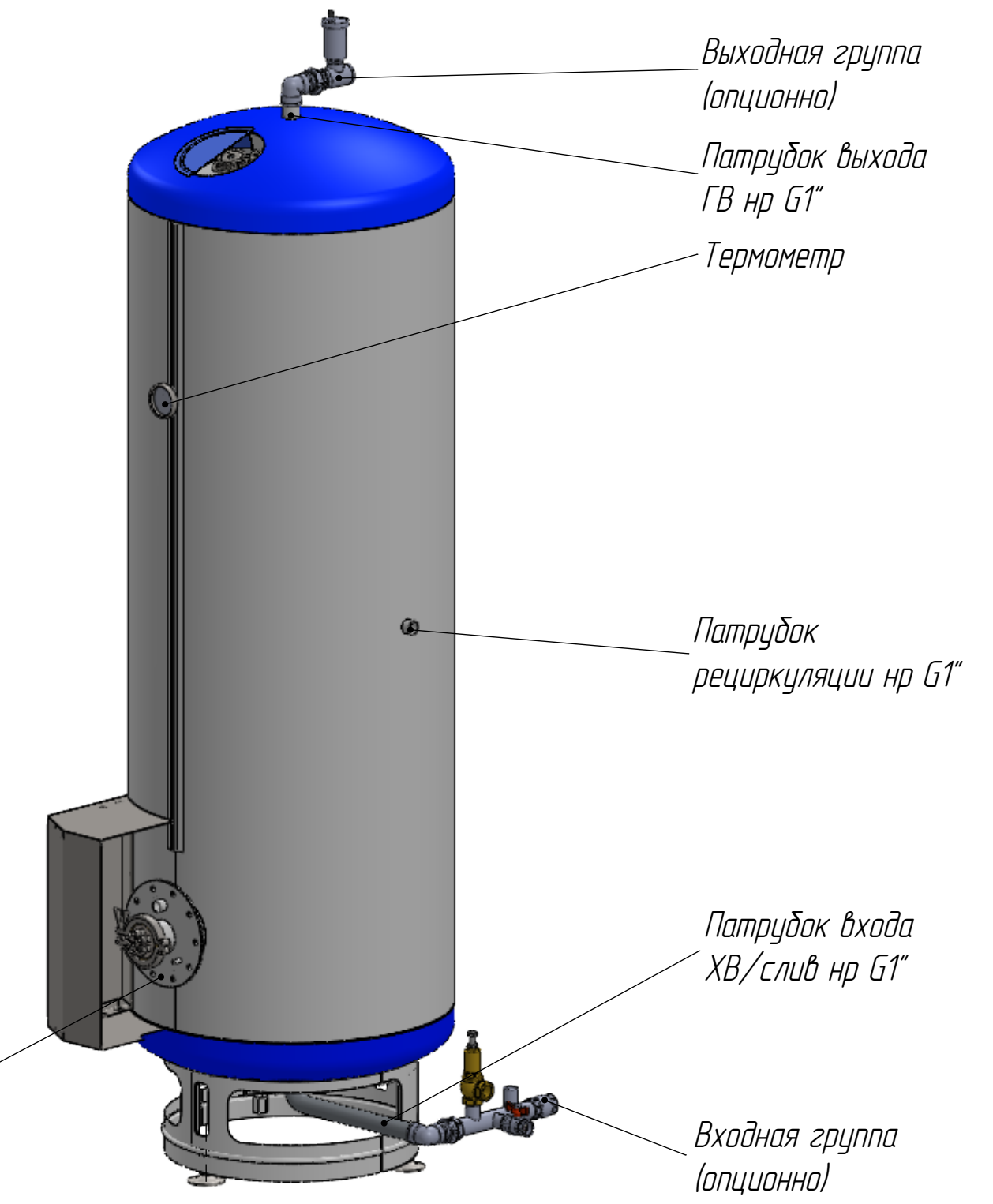
Варианты подключения водонагревателя к водопроводной сети
