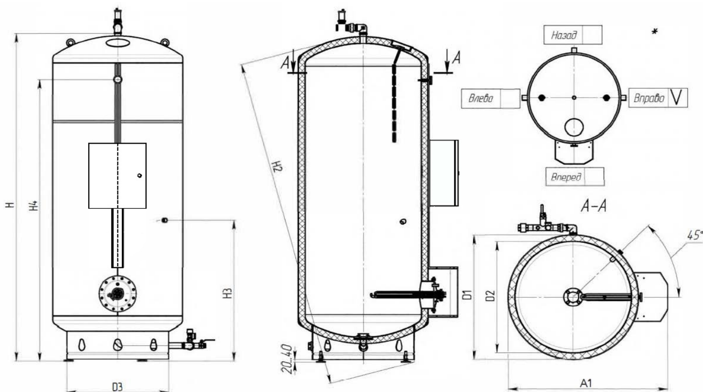
Рис. 2 Размеры основные
