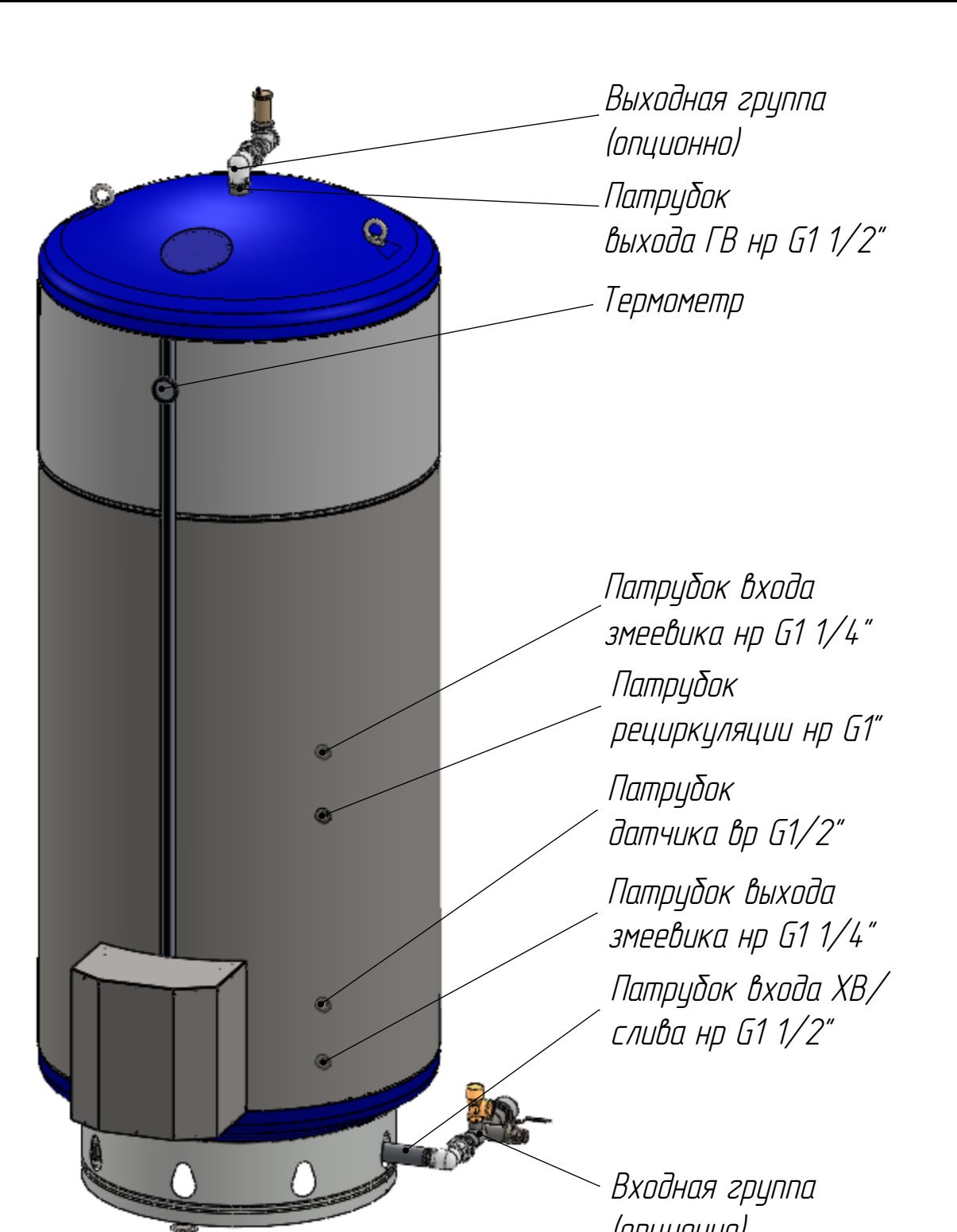
Варианты подключения водонагревателя к водопроводной сети
