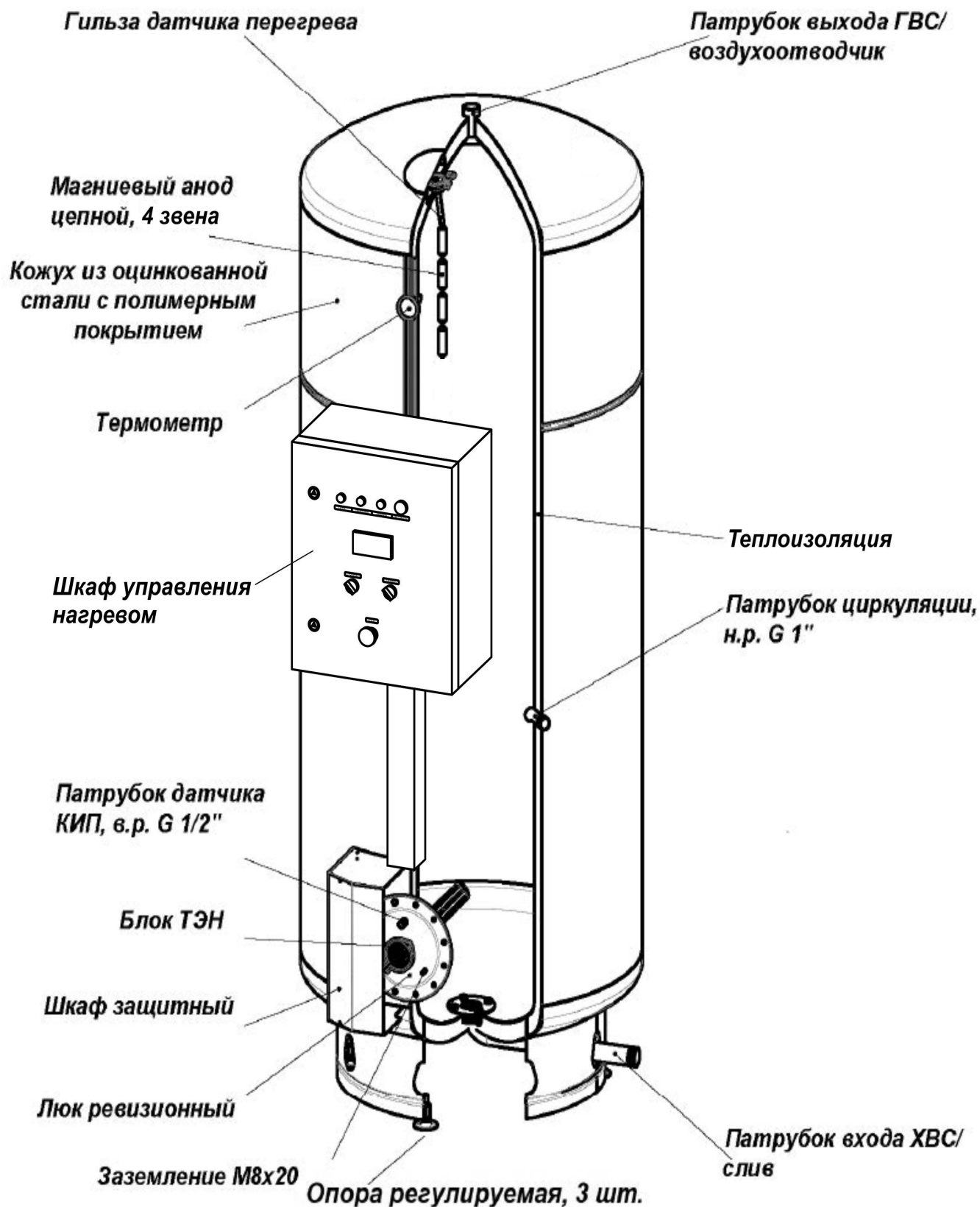
Рис. 1 Общий вид бойлера
