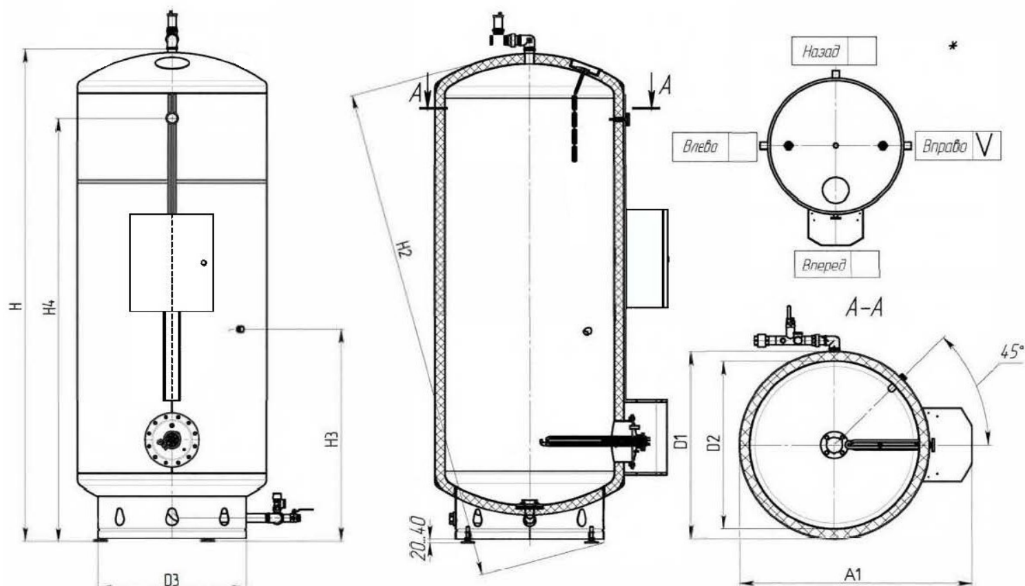
Рис. 2 Размеры основные
