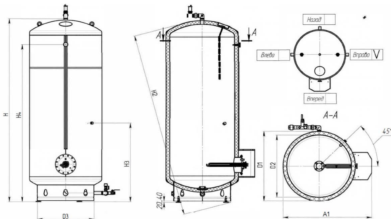
Рис. 2 Размеры основные
