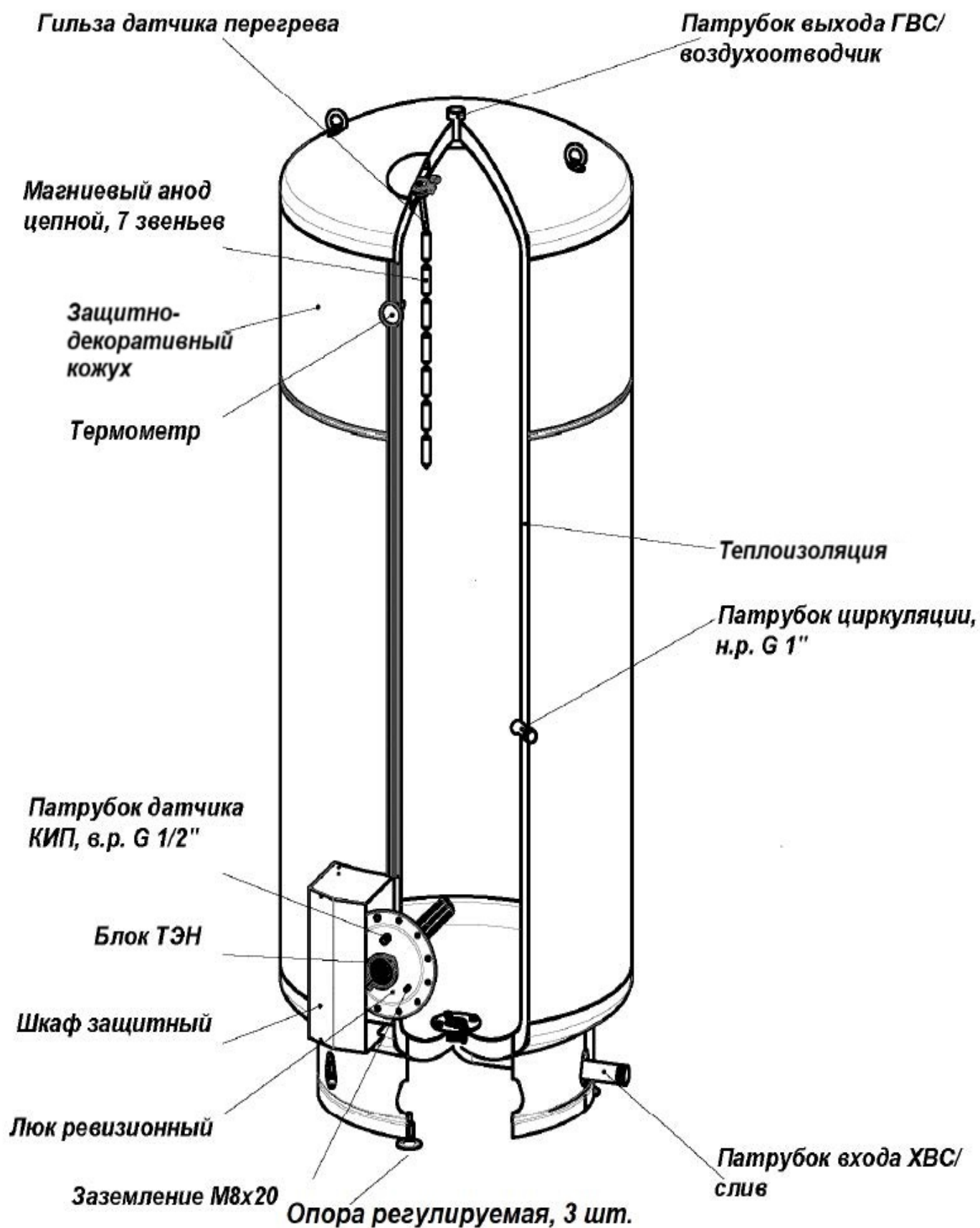
Рис. 1 Общий вид бойлера
