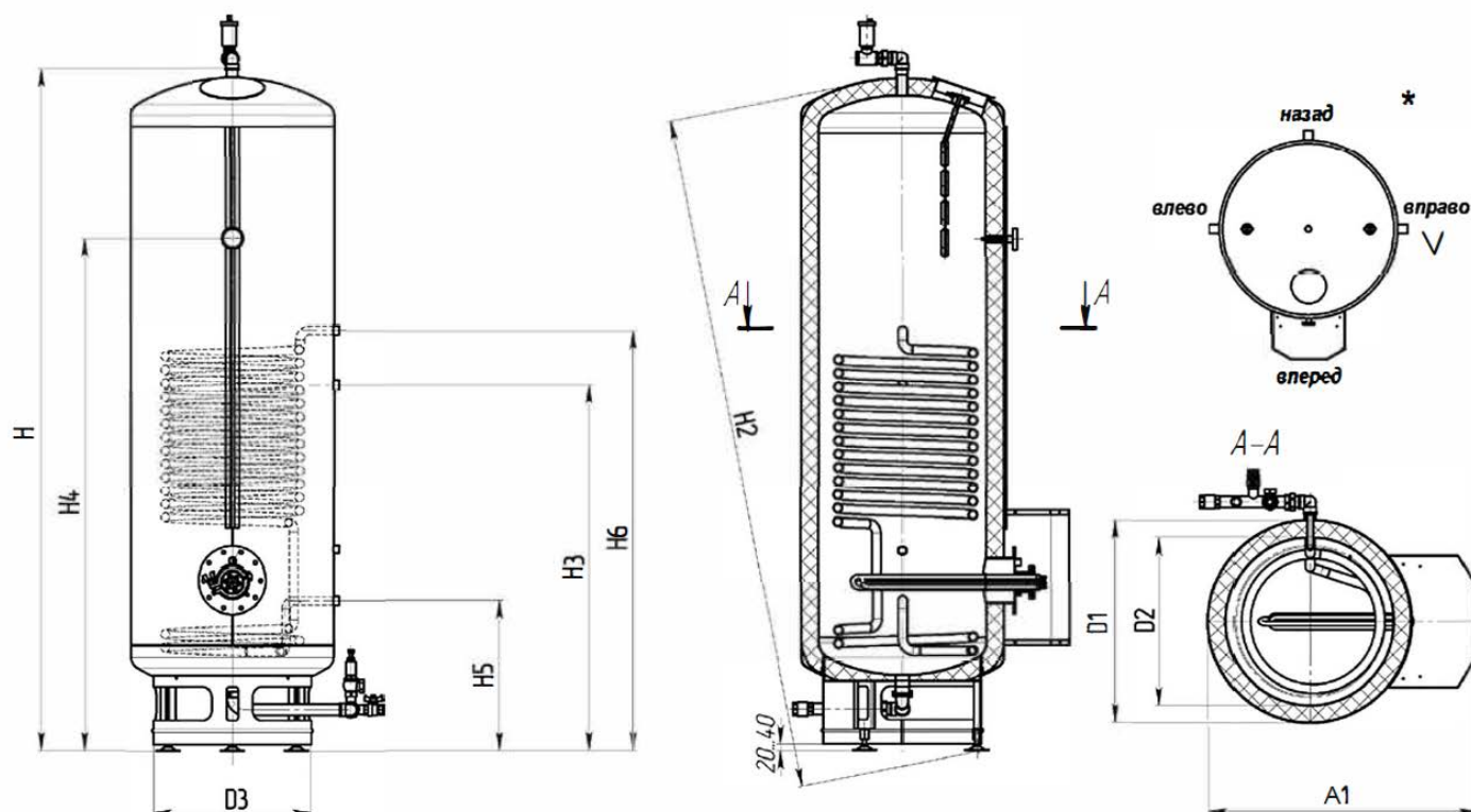
Рис. 2 Размеры основные
