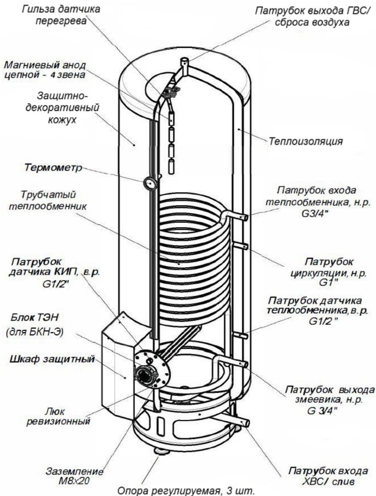
Рис. 1 Общий вид бойлера
